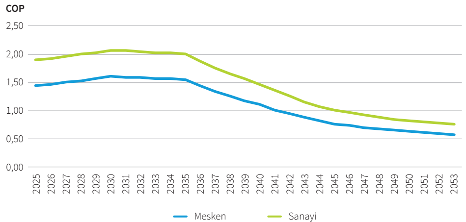
Şekil 19: Isı pompaları için eşitleyici COP değeri
