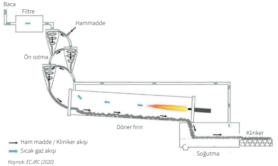
Şekil 34: Klinker üretimi
