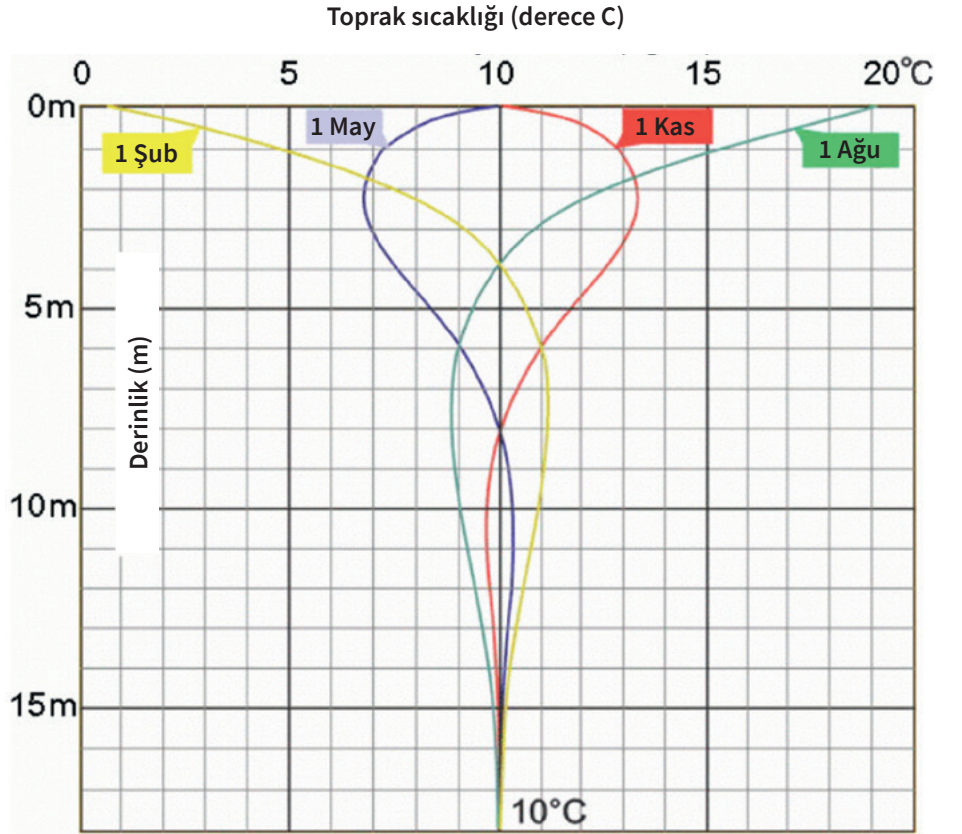
Şekil 73: Toprak derinliğine göre sıcaklık değişimi
