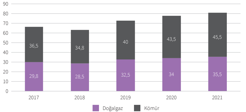
Şekil 45: Konutlarda doğalgaz ve kömürden kaynaklanan karbon emisyonları 17
