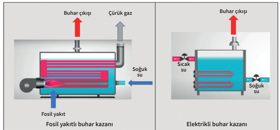
Şekil 29: Buhar / Kızgın su kazanı (Fosil yakıt ve elektrikli)
