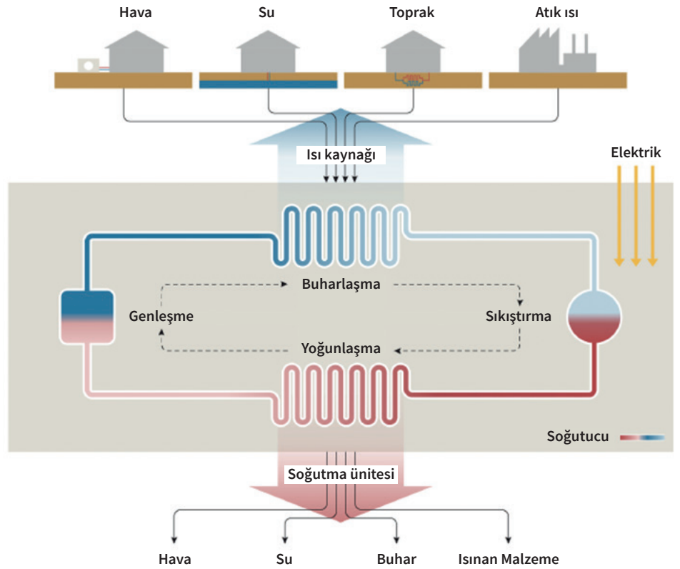
Şekil 27: Isı pompası çevrimi için akış şeması
