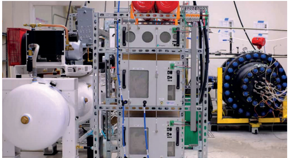
Şekil 36: Karbonsuz (Su elektrolizi) amonyak üretimi
