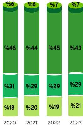
KAYNAKLARA GÖRE ENERJİ TÜKETİMİ (%)
