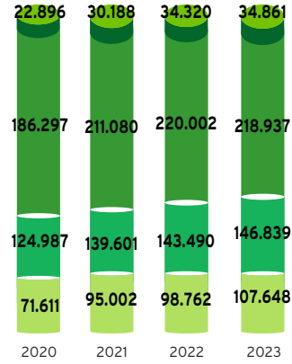
KAYNAKLARA GÖRE ENERJİ TÜKETİMİ (MWH)
