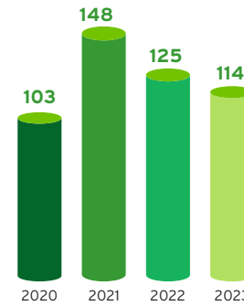
İŞLENEN SÜT BAŞINA SERA GAZI EMİSYONU (KG CO 2 e/TON)
