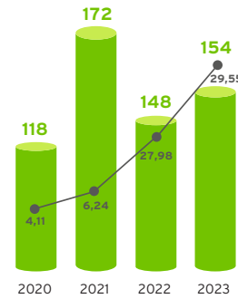
CİRO VE SERA GAZI EMİSYONU
